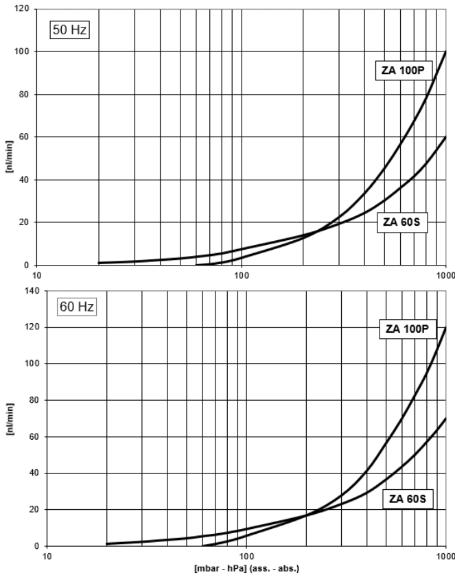
NOTA: Curve riferite alla pressione di 1013mbar (ass.) e temp. 20°C (tolleranza ±10%).
