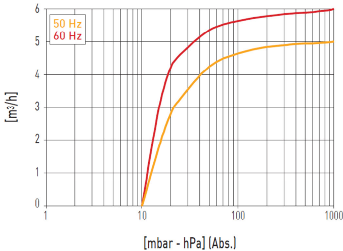
NOTE: Curve riferite alla pressione di aspirazione e temperatura 20°C (tolleranza ±10%)
