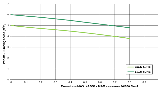
COMPRESSORE / COMPRESSOR
